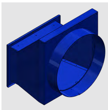
S50 Bride ø300 de refoulement d'air Art. BO19054
