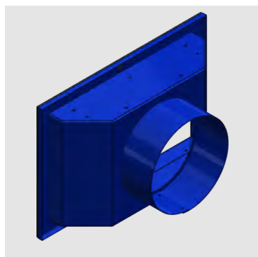
S50 Bride ø150 de refoulement d'air Art. BO19047
